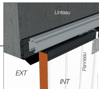
Vue intérieure Joint à lèvres (linteau)
