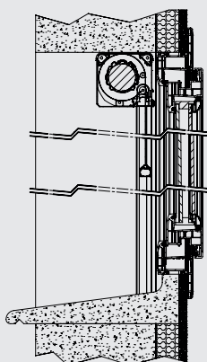
POSE AMBIO SOUS LINTEAU ENROULEMENT EXTÉRIEUR PERÇAGE TABLEAU ET DE FACE
