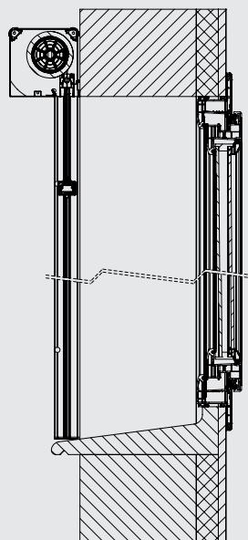
POSE AMBIO ZIP EN APPLIQUE ENROULEMENT EXTÉRIEUR PERÇAGE DE FACE
