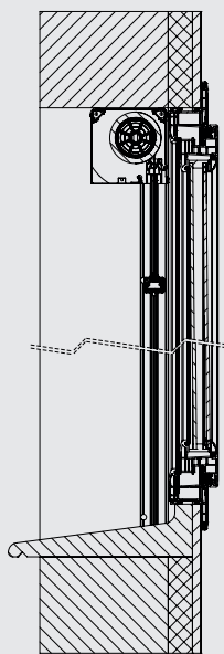
POSE AMBIO ZIP SOUS LINTEAU ENROULEMENT EXTÉRIEUR PERÇAGE TABLEAU ET DE FACE
