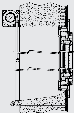
POSE AMBIO EN APPLIQUE ENROULEMENT EXTÉRIEUR * PERÇAGE DE FACE
