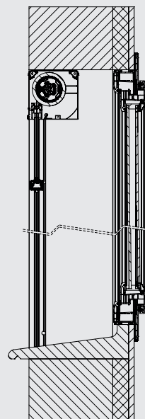
POSE AMBIO ZIP SOUS LINTEAU ENROULEMENT INTÉRIEUR * PERÇAGE TABLEAU
