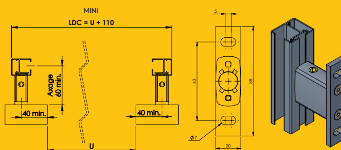
DETAILS DU SOCLE
