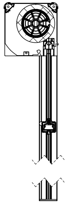
COUPE A-A
