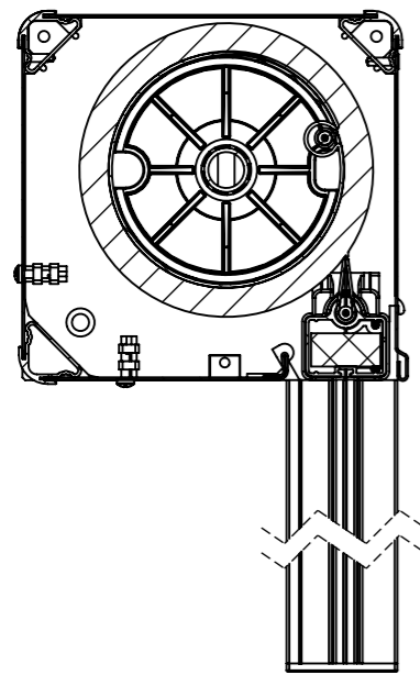
COUPE A-A
