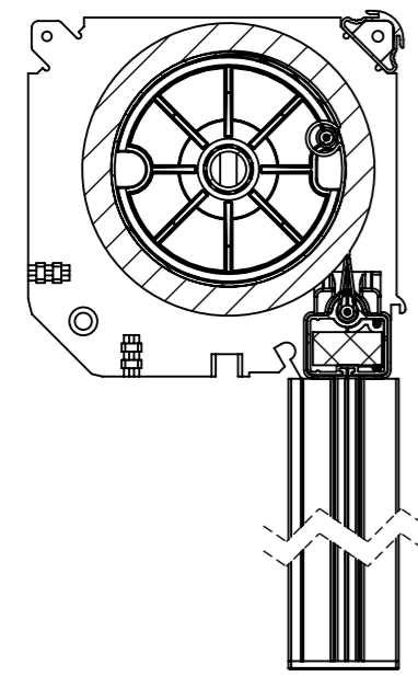
COUPE A-A
