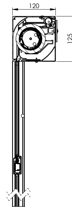
COUPE A-A
