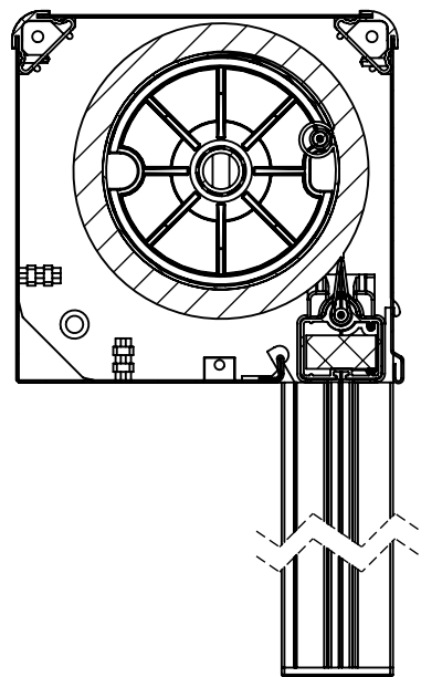
COUPE A-A
