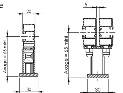
Equerre simple
