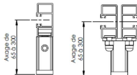
Equerre simple
